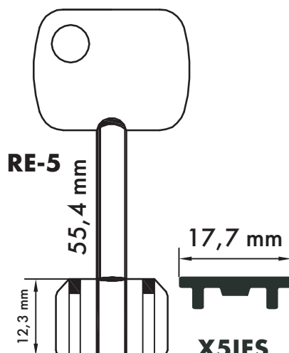
Iseo corte frontal
