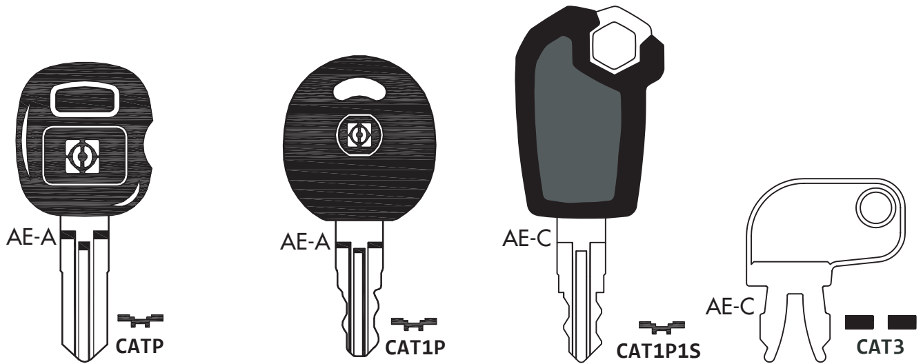
Caterpillar sin precorte Caterpillar con precorte Caterpillar 2020 Caterpillar CAT3
